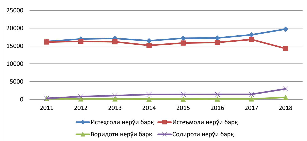
Расми 1.- Истеҳсол, истеъмол, содирот ва воридоти нуруи барқ дар соли 2018 нисбат ба моҳҳо (млрд кВт)
